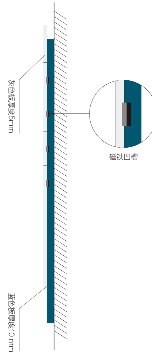
侧视图
